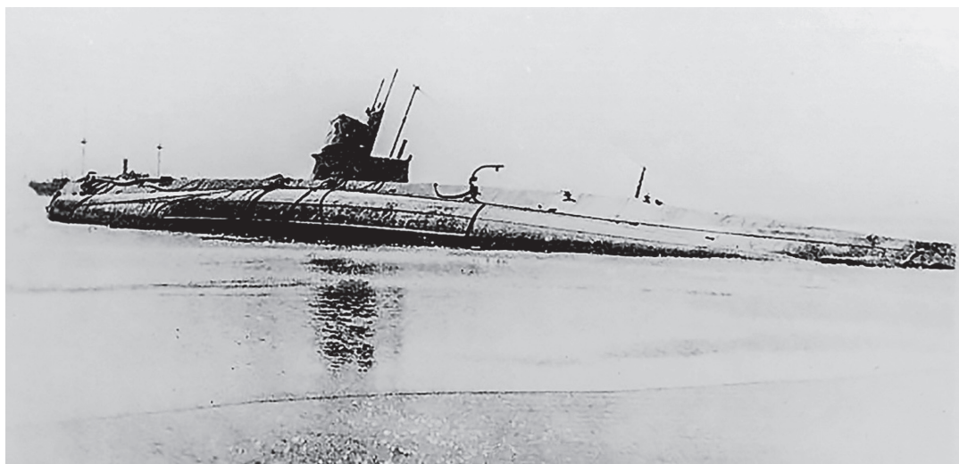
Submarino USS H-1 encallamiento en la isla Margarita, Baja California Sur, México, marzo 12 de 1920 (foto original de la colección privada de Ric Hedman).
